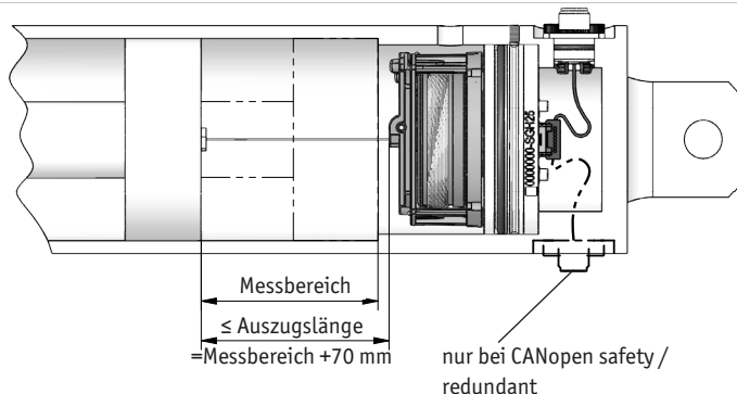
Abb. 2: Prüfung Auszugslänge
