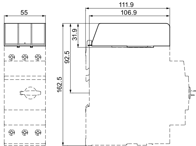
Figure C-36 3RV2938-1K
