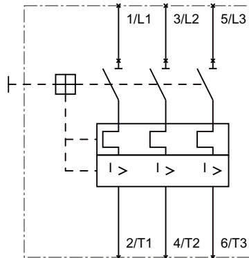
3RV10.1-...0
