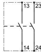
3RV2901-.F
